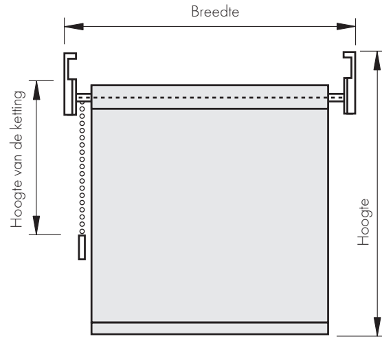
Plafondbevestiging
